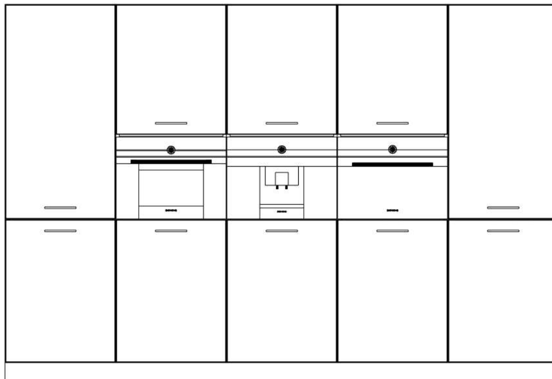
Vooraanzicht Kastenwand.
